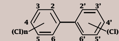
PCB : formule développée
